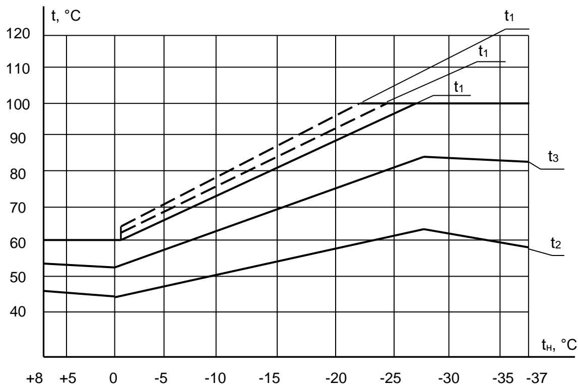
Температурный график ТЭЦ МУП «ЯТЭК» 115 – 70 °С со срезкой до 100 °С.
